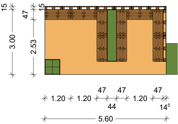
Grundriss M=1:00
